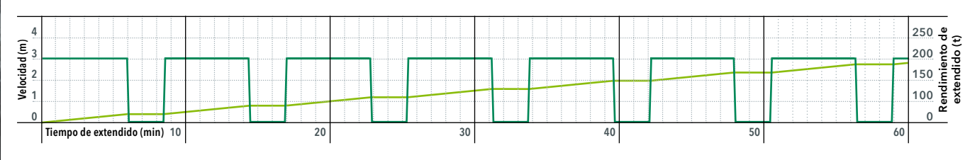
Extendido con VÖGELE PowerFeeder (indicación en m/min)
